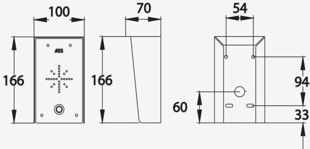
SLIM - IMPERIAL NON KP
